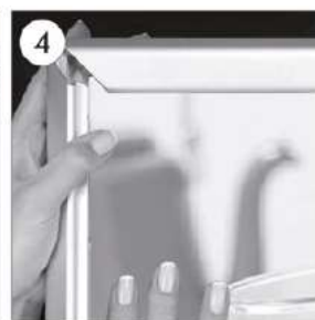
4 Sæt frontpladen i og luk profilerne
